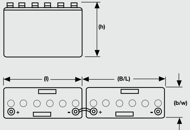
12V 1 OPzS 50 LA - 12V 3 OPzS 150 LA
