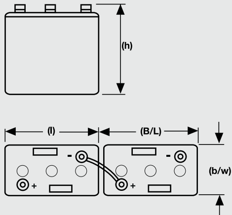
6V 4 OPzS 200 LA - 6V 6 OPzS 300 LA
